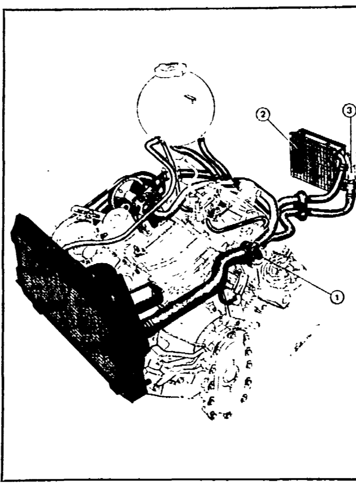
La Peugeot 104 GL6 fotografata con il portellone posteriore aperto. Nel disegno qui sopra lo schema del circuito di raffreddamento...
