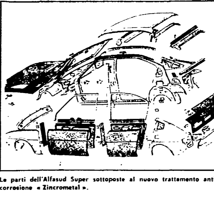
Le parti dell'Alfasud Super sottoposte al nuovo trattamento anticorrosione «Zincrometal».
