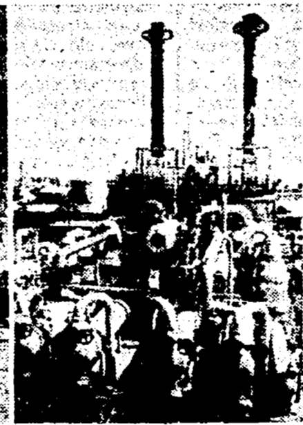
e quindi stirolo
