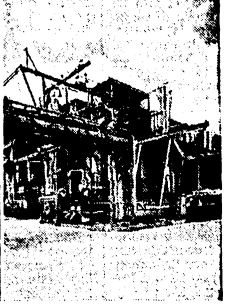
che tra l'altro dà luogo a polietilene;
