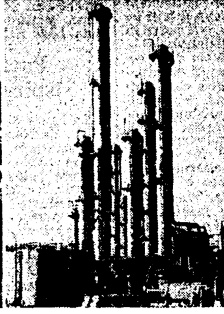
cumene, che dà fenolo e acetone,
