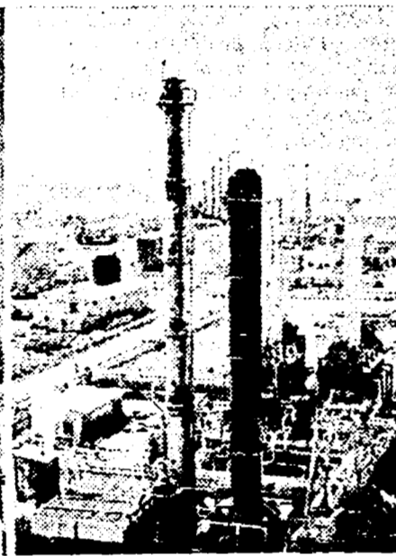
dal quale derivano ammoniaca
