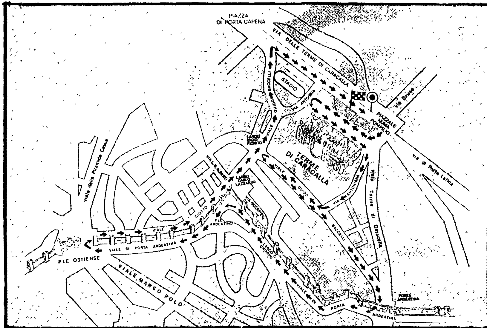
La planimetria del G.P. della Liberazione che si disputerà oggi sul circuito di Caracalla - Porta San Paolo con inizio alle ore 13,30. Il circuito misura Km. 5,300 e dovrà essere ripetuto 23 volte per complessivi 121,900 chilometri. L'arrivo è previsto per le ore 16,40
