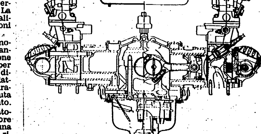
Il boxer AlfaSud che equipaggia i due modelli Sprint Veloce visto in sezione sulla bilia...
